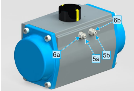
Fig. 6-3 Einstellung des Schwenkantriebs bar-agturn
