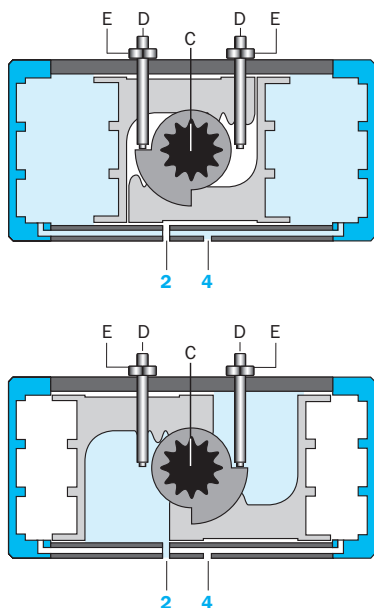
Fig. 3-6 Rotary actuator bar-acturn function „double-acting“ GD-032 till 210
