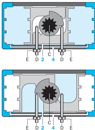
Fig. 3-7 Rotary actuator bar-acturn function „double-acting“ GD-240 till 400
