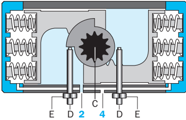
Fig. 3-9 Rotary actuator bar-actuator function „single-acting“ GS-240 till 400
