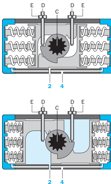
Fig. 3-8 Rotary actuator bar-acturn function „single-acting“ GS-052 till 210
