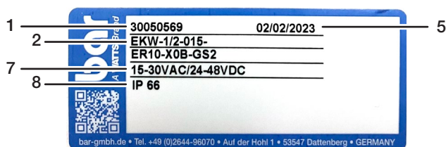
Abb. 3-2 Typenschild EKW
