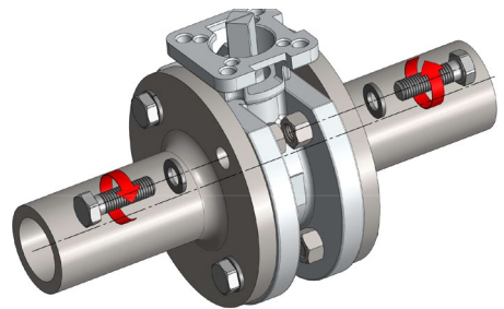
Fig. 5-1 Montage Kugelhahn in eine Rohrleitung
