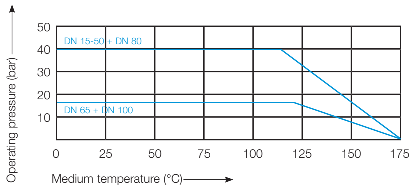
Fig. 14-1 Druck-Temperatur-Diagramm
